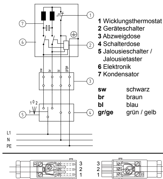
Fig. 5 Schaltbild RolTop 230 V / 50 Hz und Kabelbelegung bei Verwendung mit Hirschmann-Steckverbindung STAS-3
